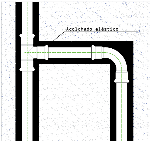
Bajo enlucido
