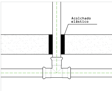
Bajo galería
